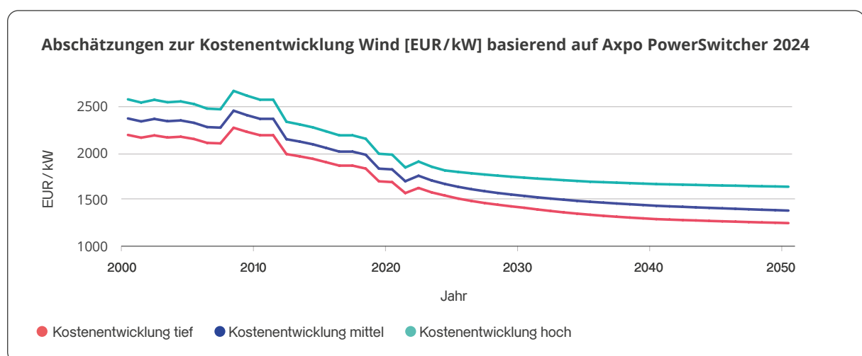
Abbildung 2: Die durchschnittlichen Kosten pro kW installierter Kapazität sind bei Wind in Deutschland in den letzten Jahrzehnten erheblich gefallen. Daten: real bei 2024-Werten, 1990–2023 historische Daten DE (umgelegt auf Preisniveau CH), 2024–2050 angenommene Entwicklung CH. Quelle: Axpo Power Switcher.
